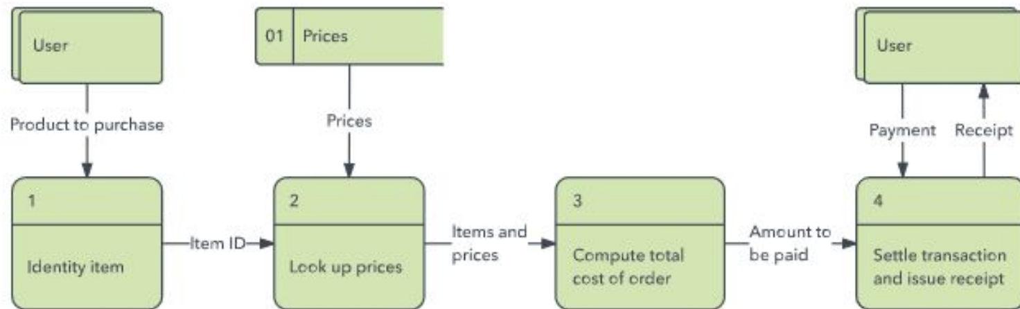
Logical DFD
